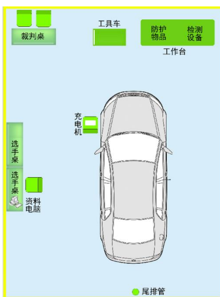
图 1 整车竞赛工位布置图
