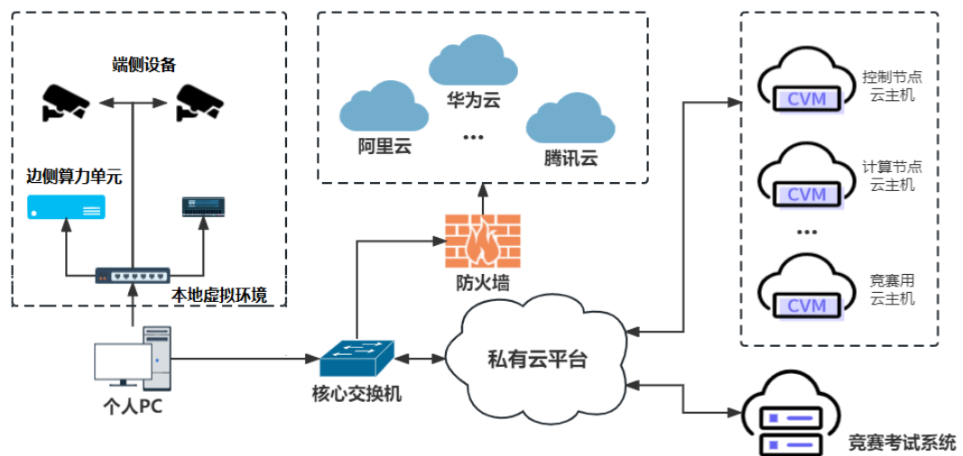
图 1 系统架构图
