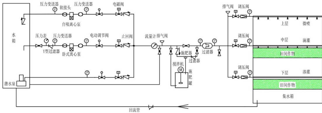
图 1 智能节水系统安装与运维平台布置图
