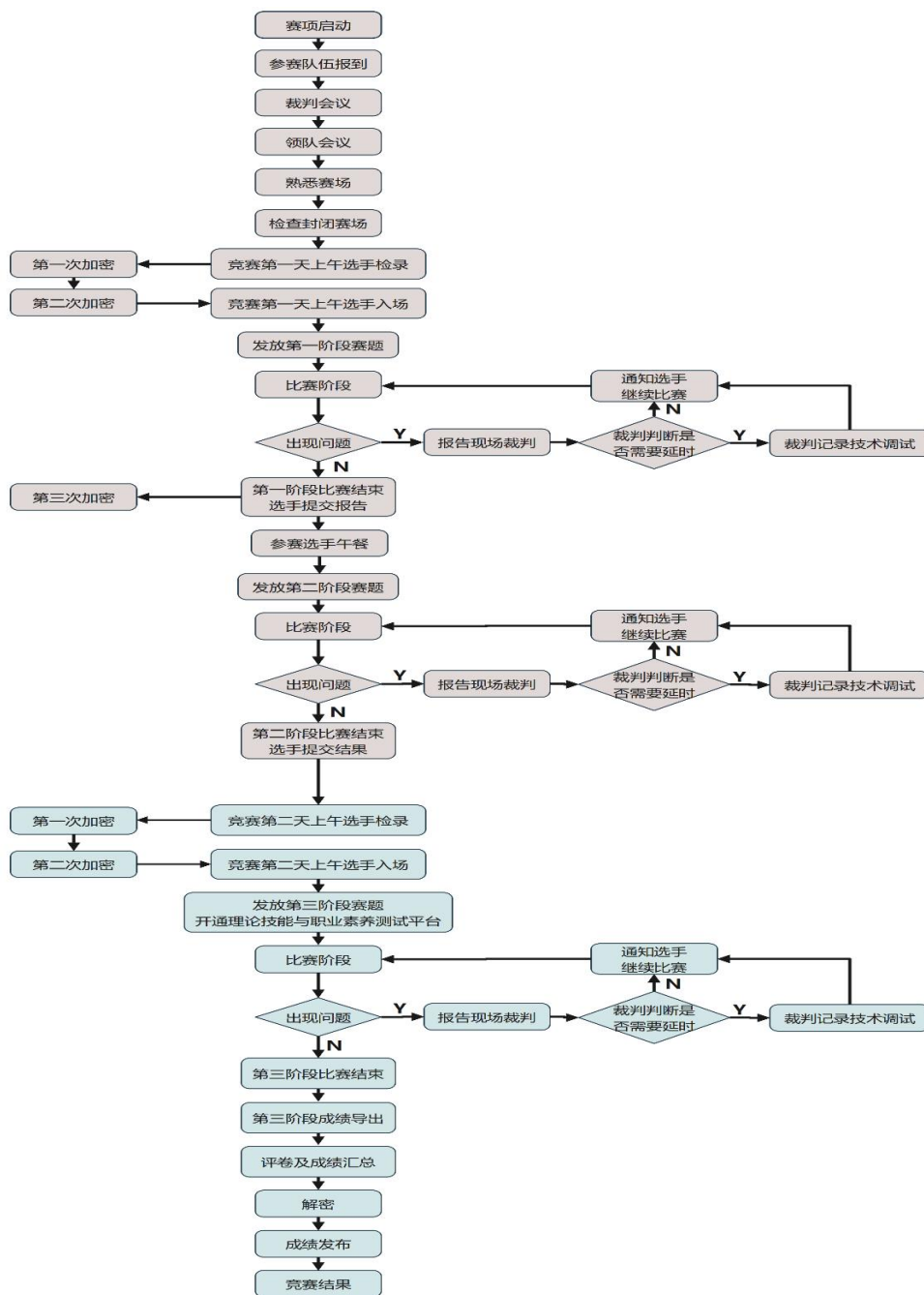
图 1 竞赛流程图
