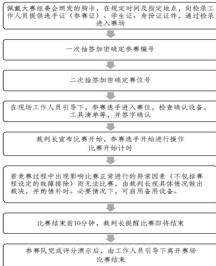
图1 竞赛流程图
