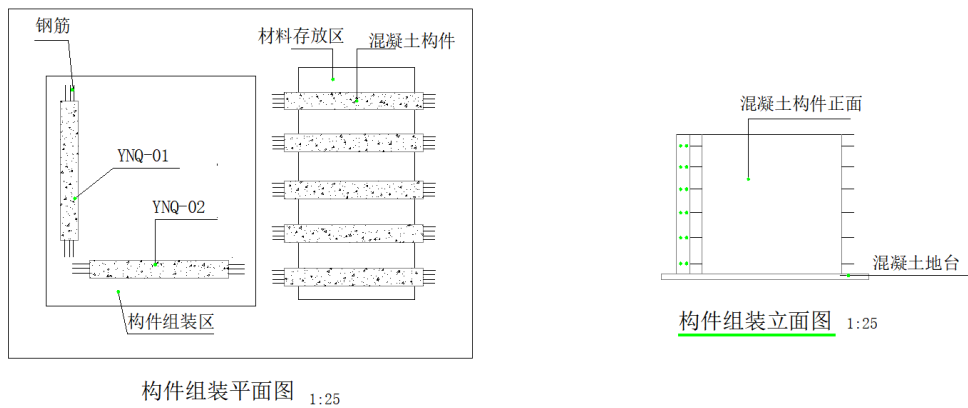
图 1 构件组装图
